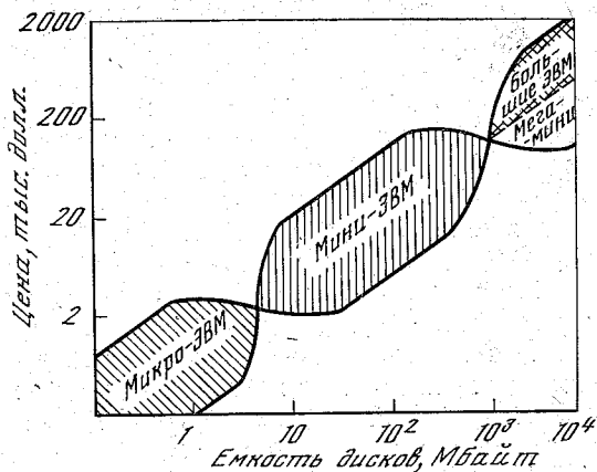
Рис. 12. Классификация малых ЭВМ
